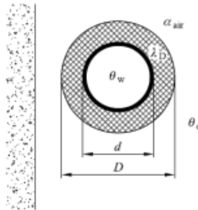
Figura C.2 - Tubazione isolata corrente in aria
